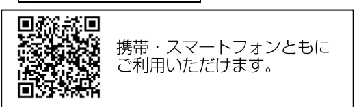
図3 QRコード
