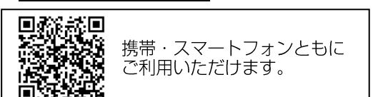
図3 QRコード
